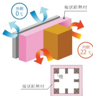
サーラの壁外断熱工法
