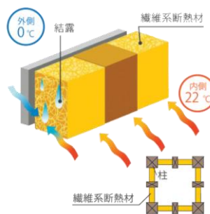
一般的な充填断熱工法
